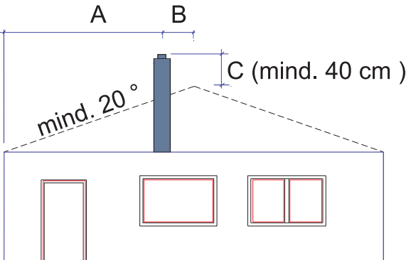
Abb. 2: Flachdach; fiktiver First mit mind. 20° und A > B und C > B
