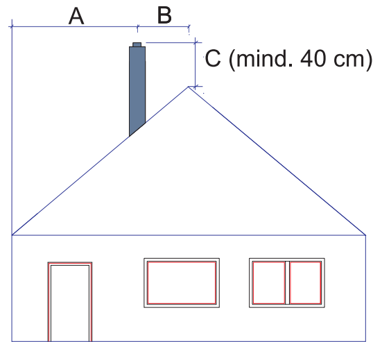
Abb. 1: A > B und C > B
